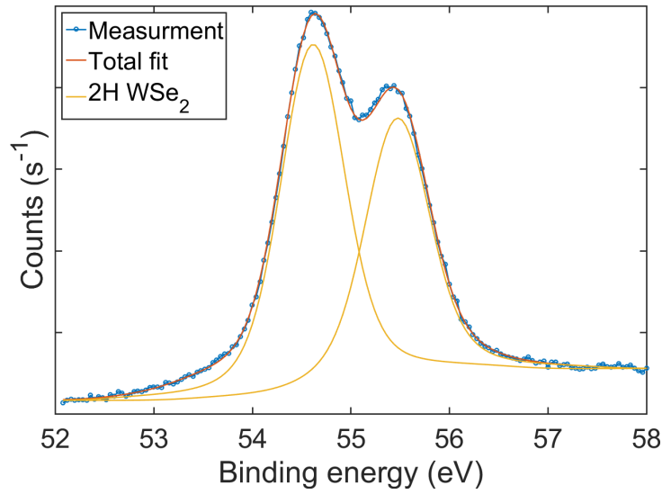
(b) Se 3d
