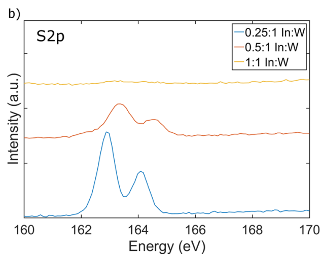
(b) S 2p
