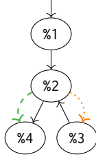
Fig. 5. The “do while false” idiom
