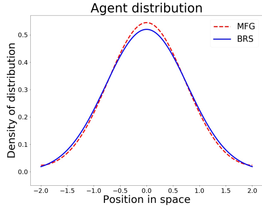
(D) \beta = 1, \frac{\sigma^2}{2} = 0.2
