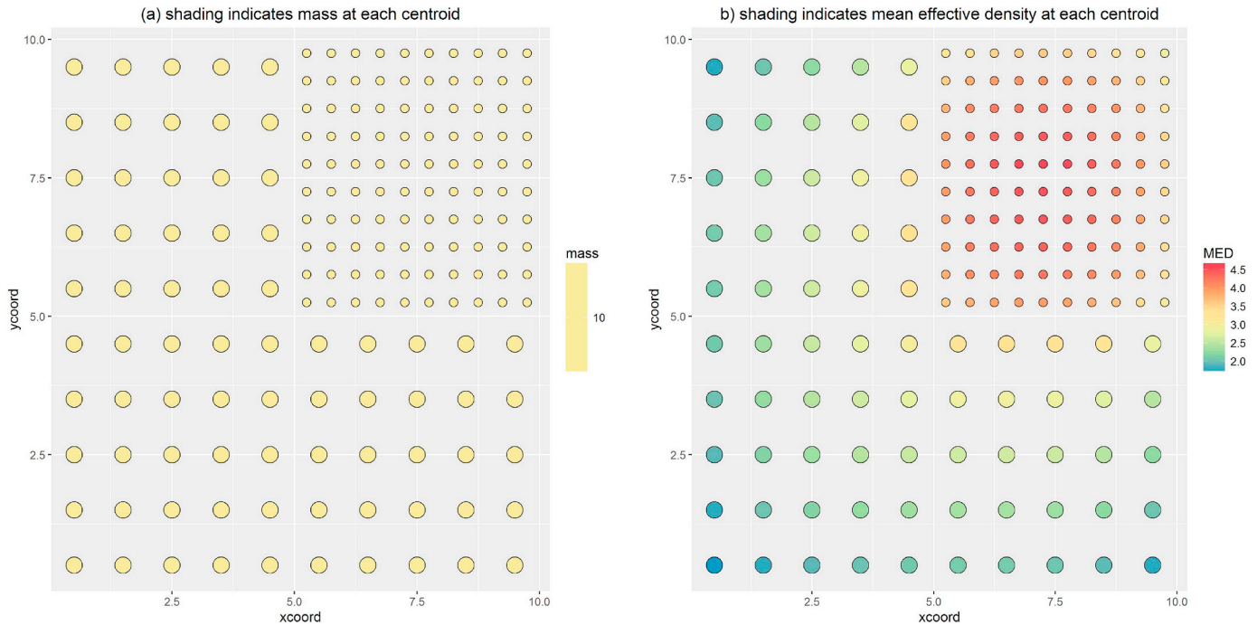
Fig. 4. MED values for zones of variable size.
