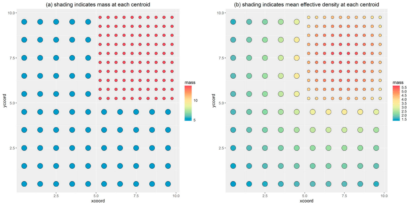
Fig. 5. MED values for zones of variable size and mass.
