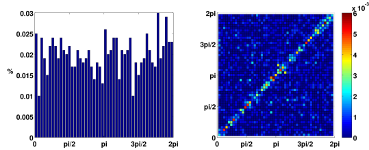
(d) N = 10^5
