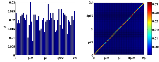
(d) N = 10^5
